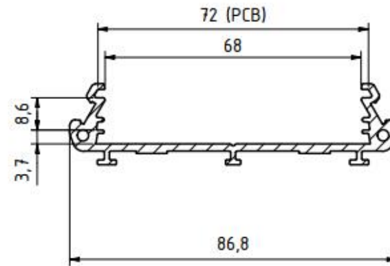
A-A ( 1 : 1 )
